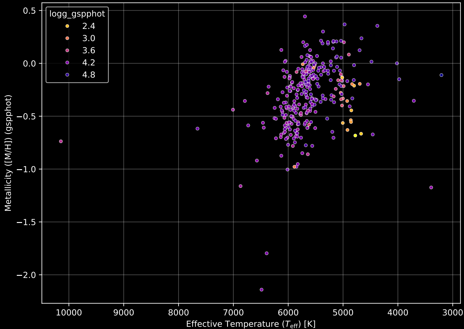
GALAH DR4 Field: [6892] Stellar Population Parameters (n= 303)
